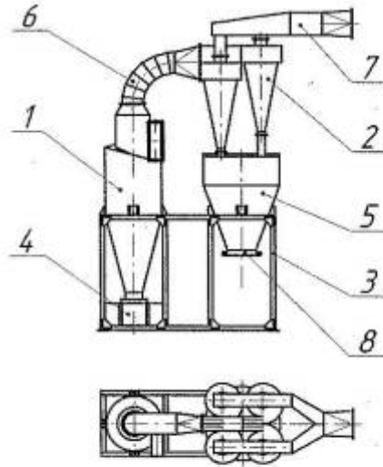
Рис.1 Установка циклонов ПКП-229
